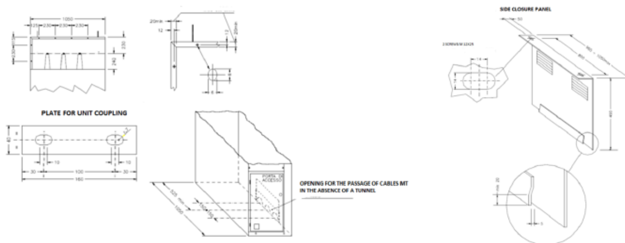
Figura 75 – Panou de închidere laterală
