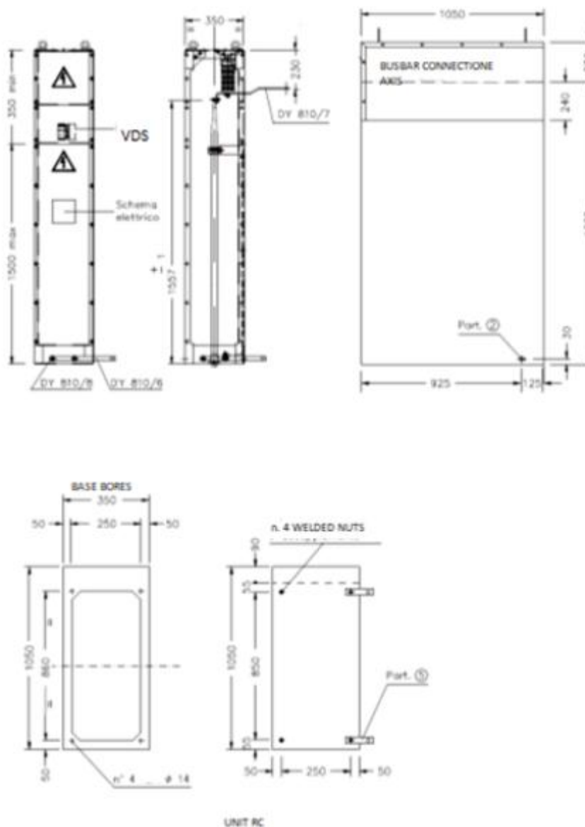
Figura 65 - CELULA RC
