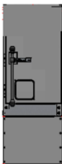
Figura 53 – Plasarea manetei de comandă pe ușa compartimentului pentru cabluri
