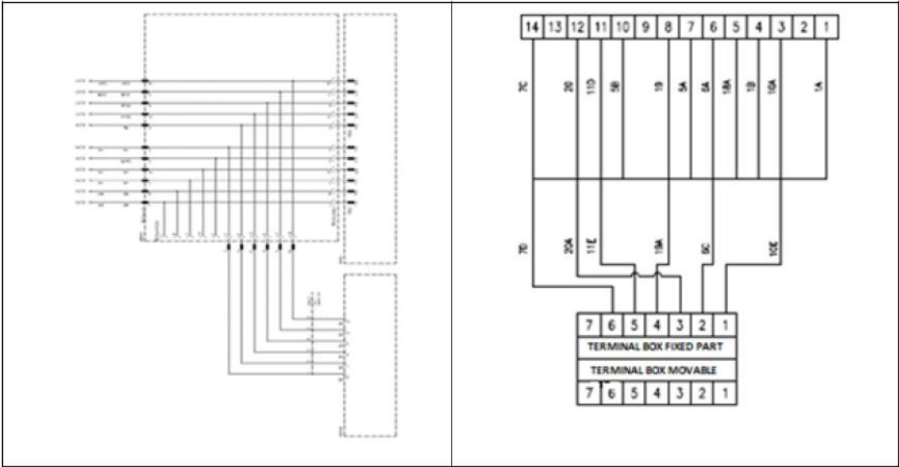
Figura 11 – Schema electrică
