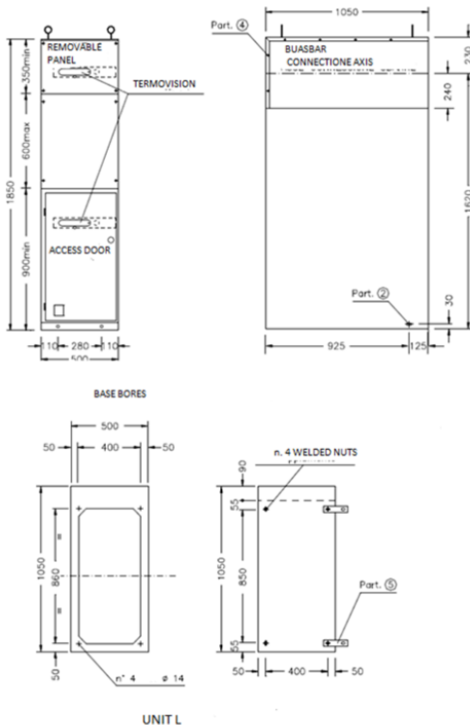
Figura 66 - Dimensiunile CELULEI L
