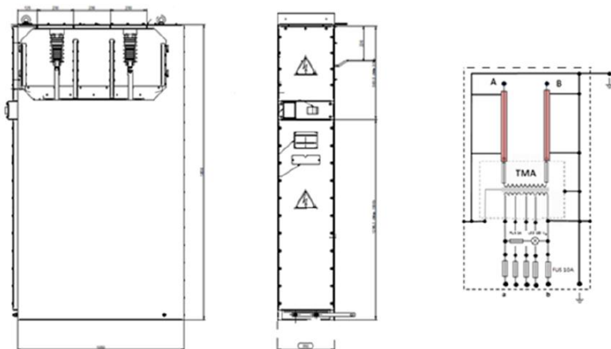
Figura 30 – Celula tip transformator autoprotejat
