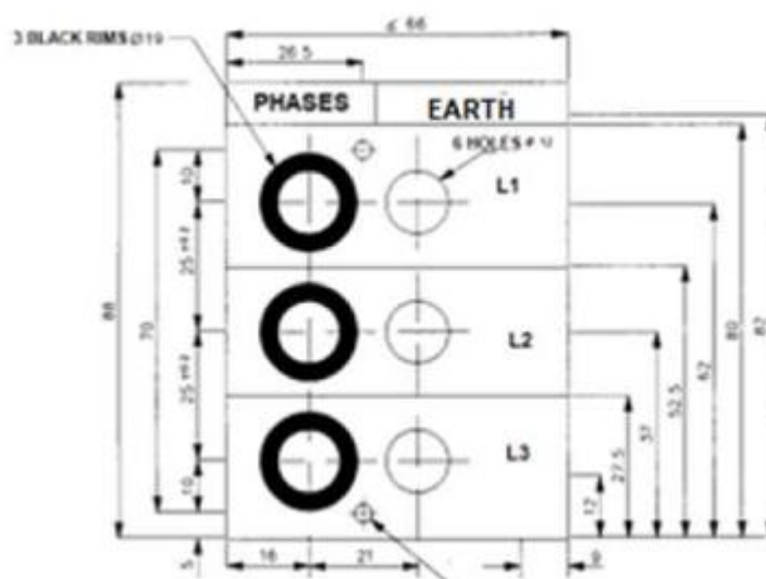
Figura 81 – Parte fixă
