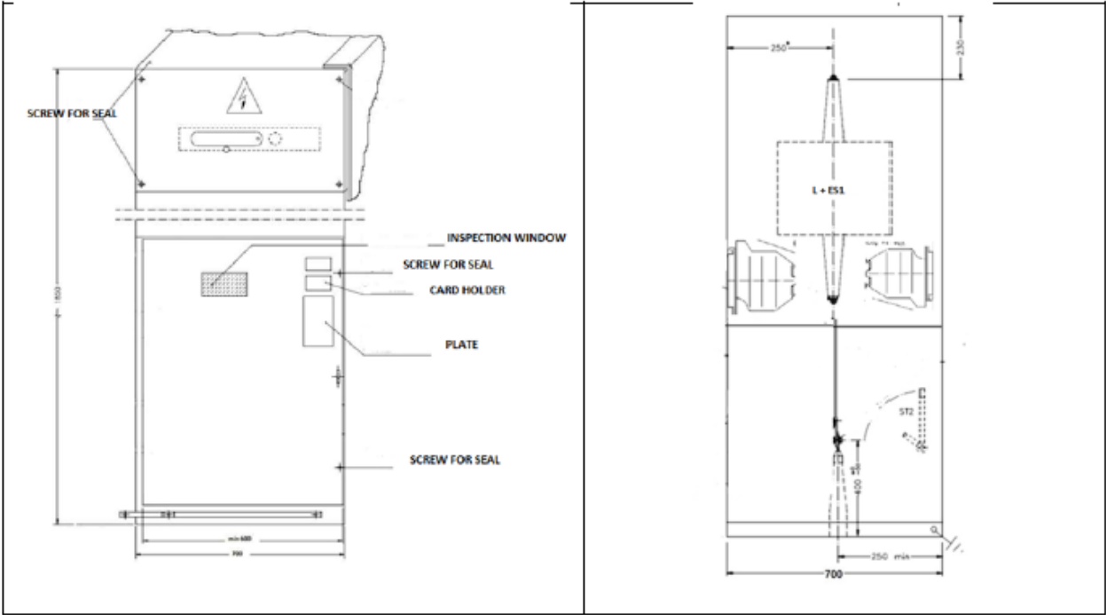
Figura 73 – Celula M - vedere frontală
