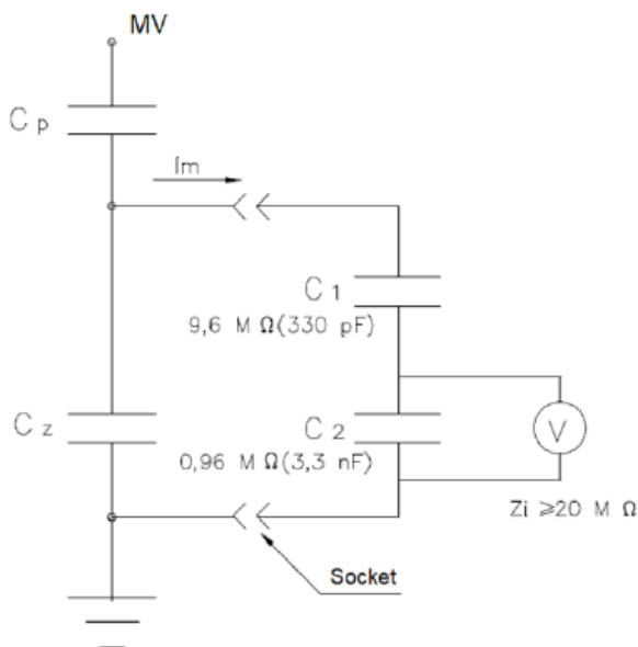
Figura 84 – Aranjament de testare
