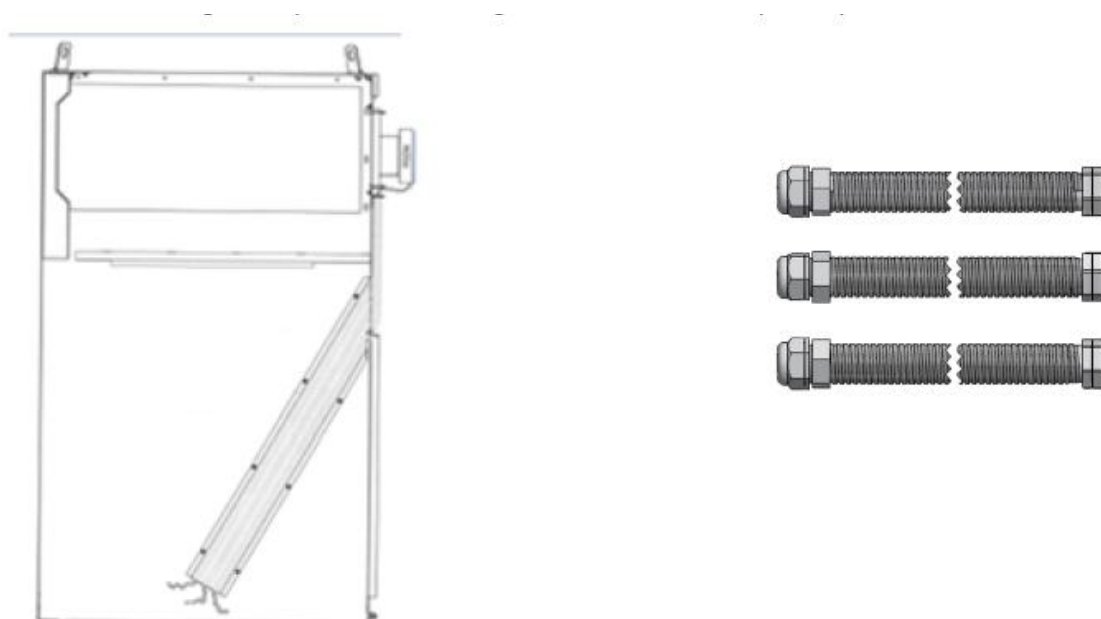
Figura 48 – Compartiment pentru cabluri
