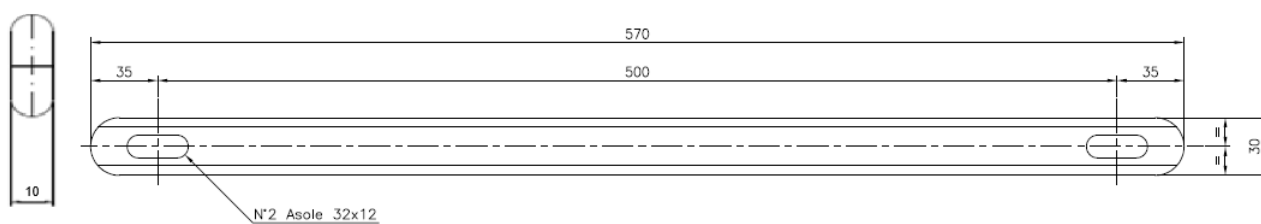
Figura 78 – bară de cupru 570 mm
