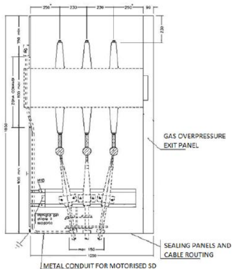
Figura 67 - Dimensiuni interne ale celulei L
