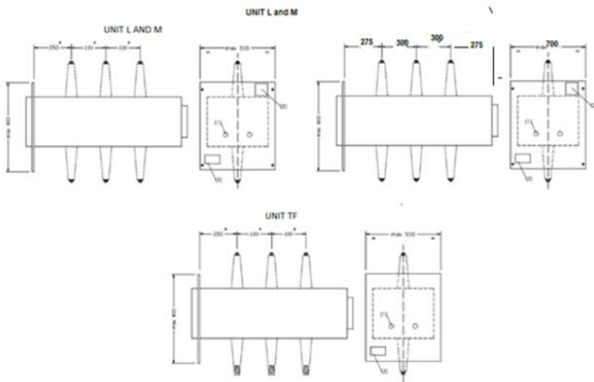
Figura 76 - Izolatoare de distanță pentru celulele L și M
