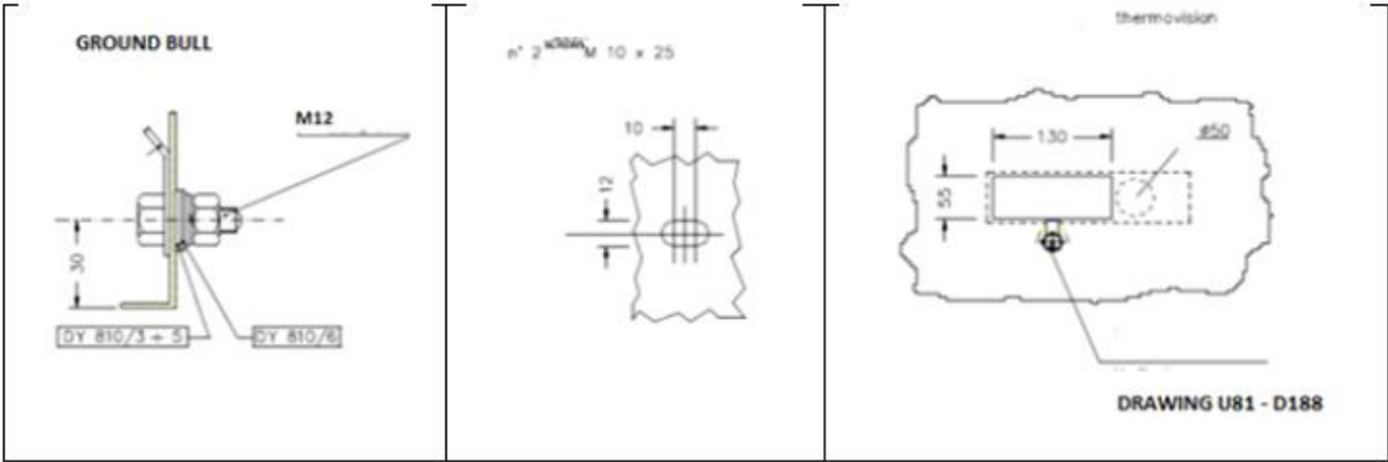
Figura 74 - Conexiune la legare la pământ
