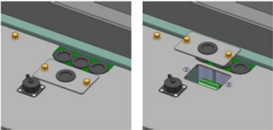
Figura 10 - Bloc terminal
