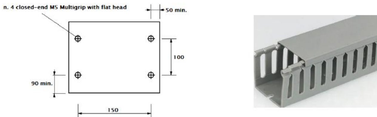
Figura 58 - Suport pentru dispozitivul de detectare a defectelor și conducta de cablu
