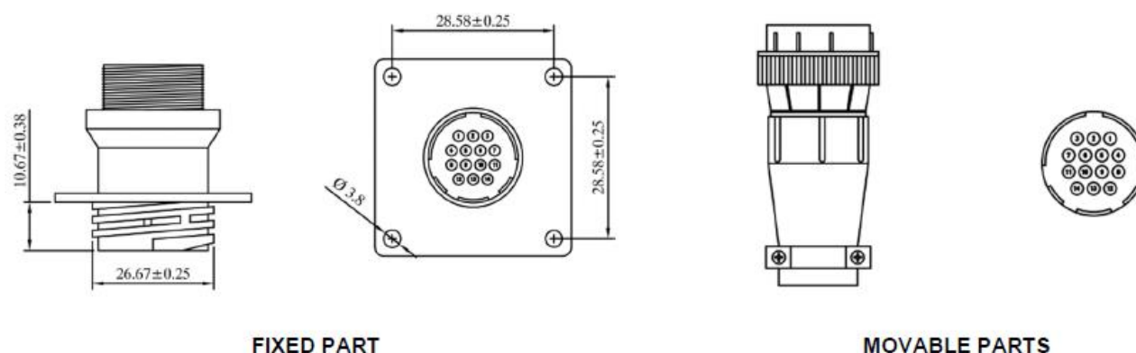
Figura 59 - Conectori
