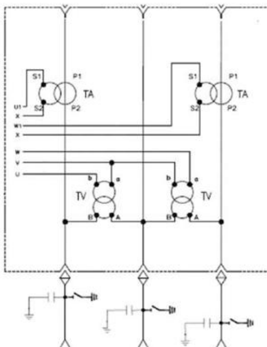
Figura 41 – Scheme de conectare
