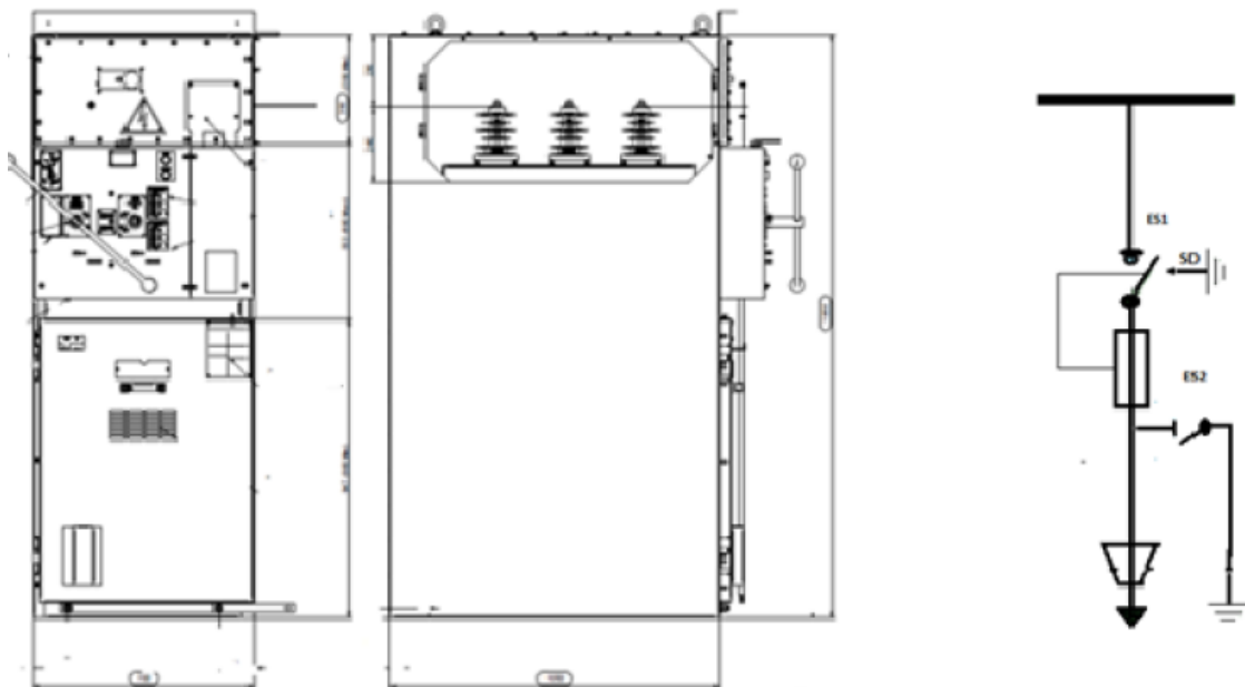
Figura 18 - Celula de protecție a transformatorului
