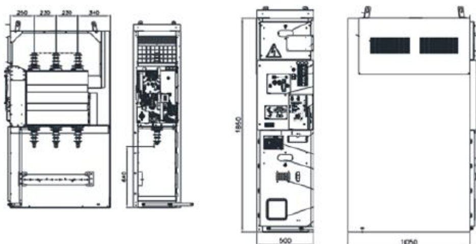
Figura 61 - CELULA CBL TIP A
