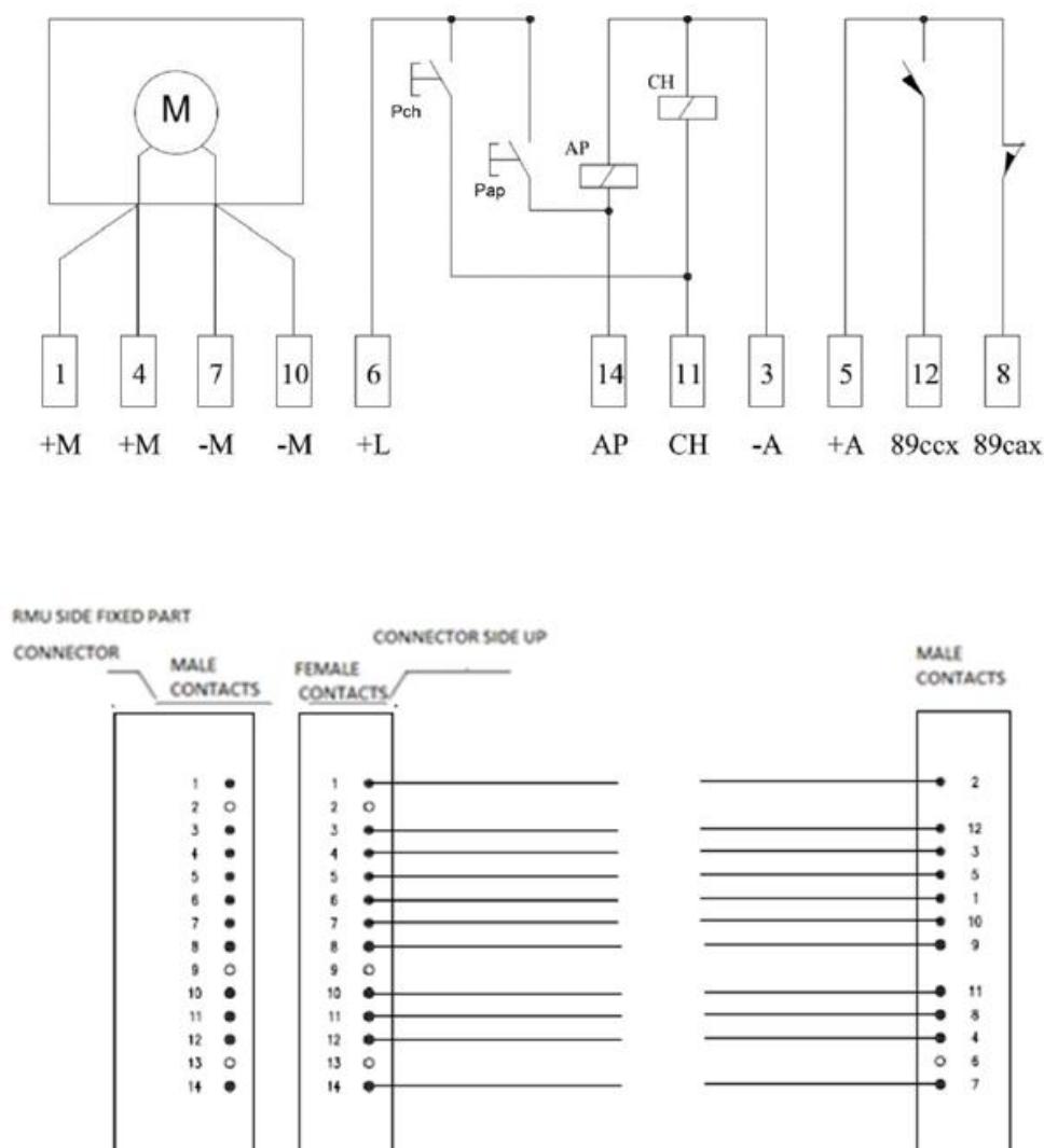
Figura 60 - Schema electrică a comenzii IMS
