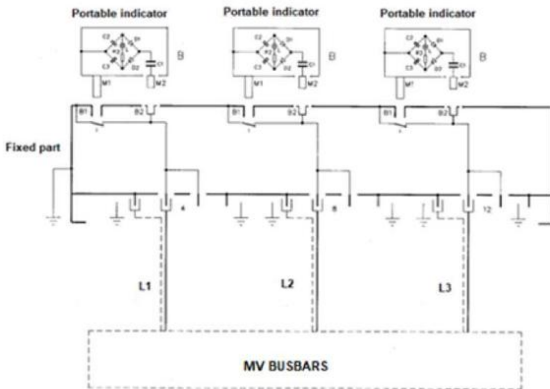
Figura 82 – Schema electrică
