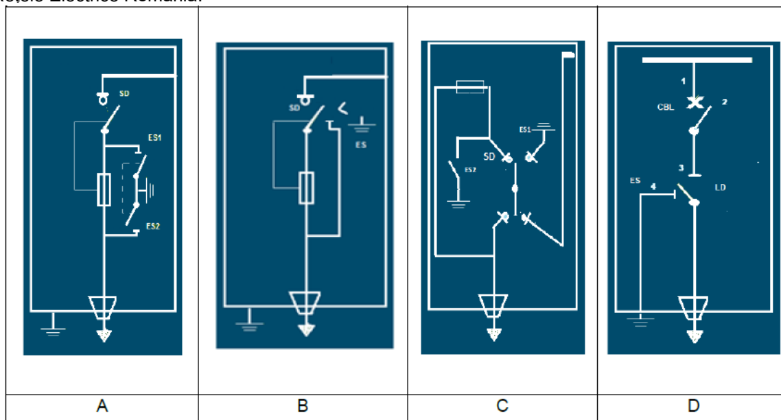
Figura 2 – Schemă monofilară celula de protecție trafo
