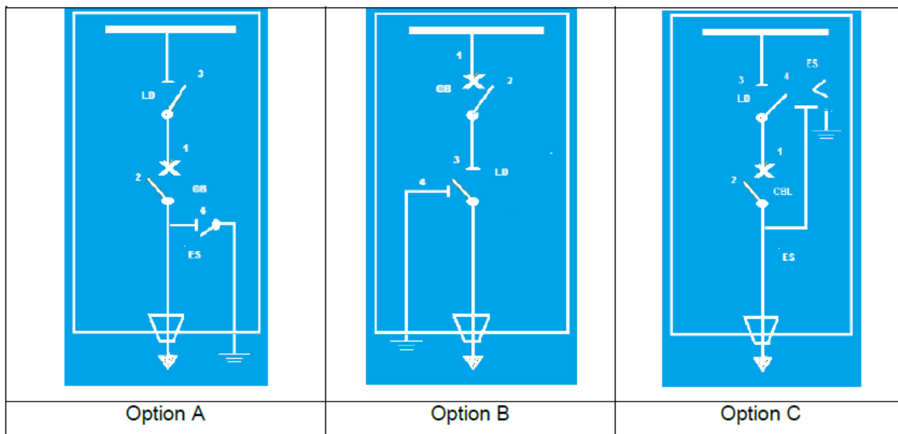
Figura 1 – Schemă monofilară celula de linie cu întrerupător
