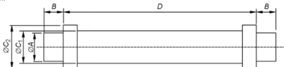
Figura 25 – Dimensiunile siguranței
