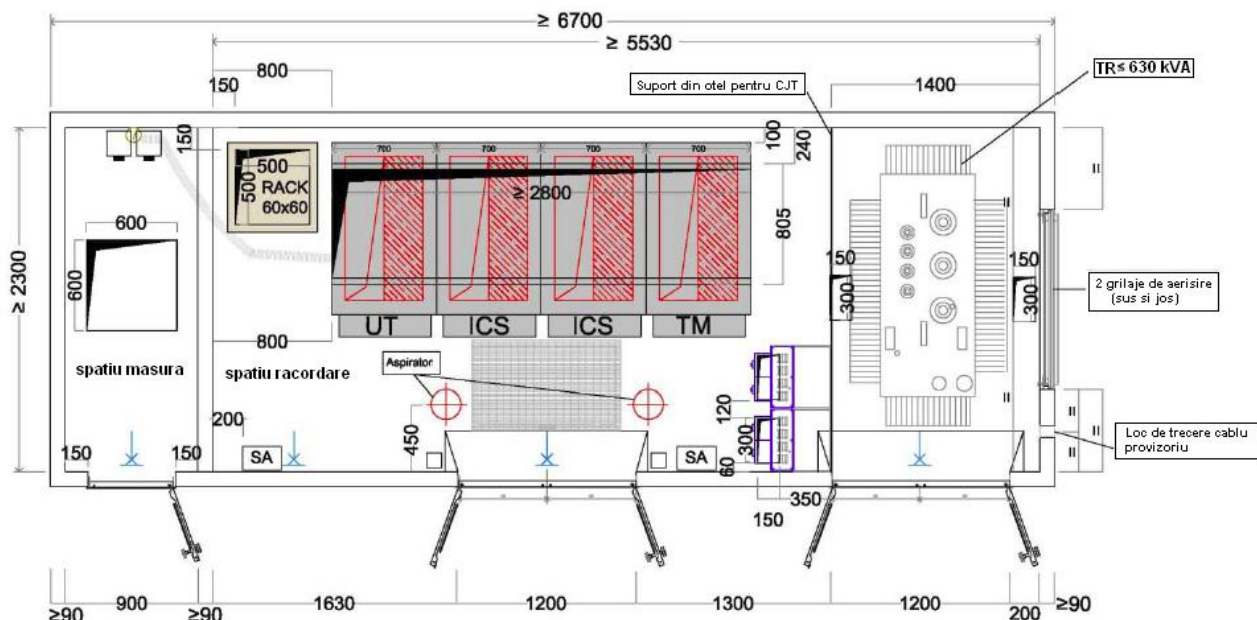
Figura 1 - Plan post de transformare și racordare Utilizator
