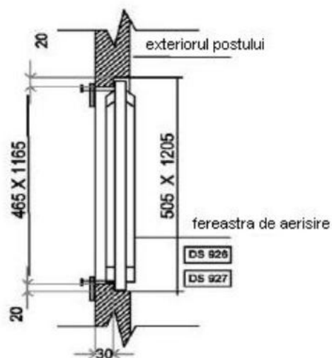
SECȚIUNE F-F
