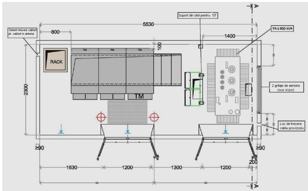
Figura – 1. - Dimensiunile postului si schema de funcționare
