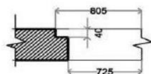
SECȚIUNE G-G
