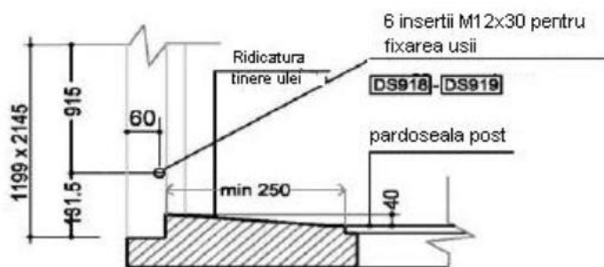
SECȚIUNE F-F
