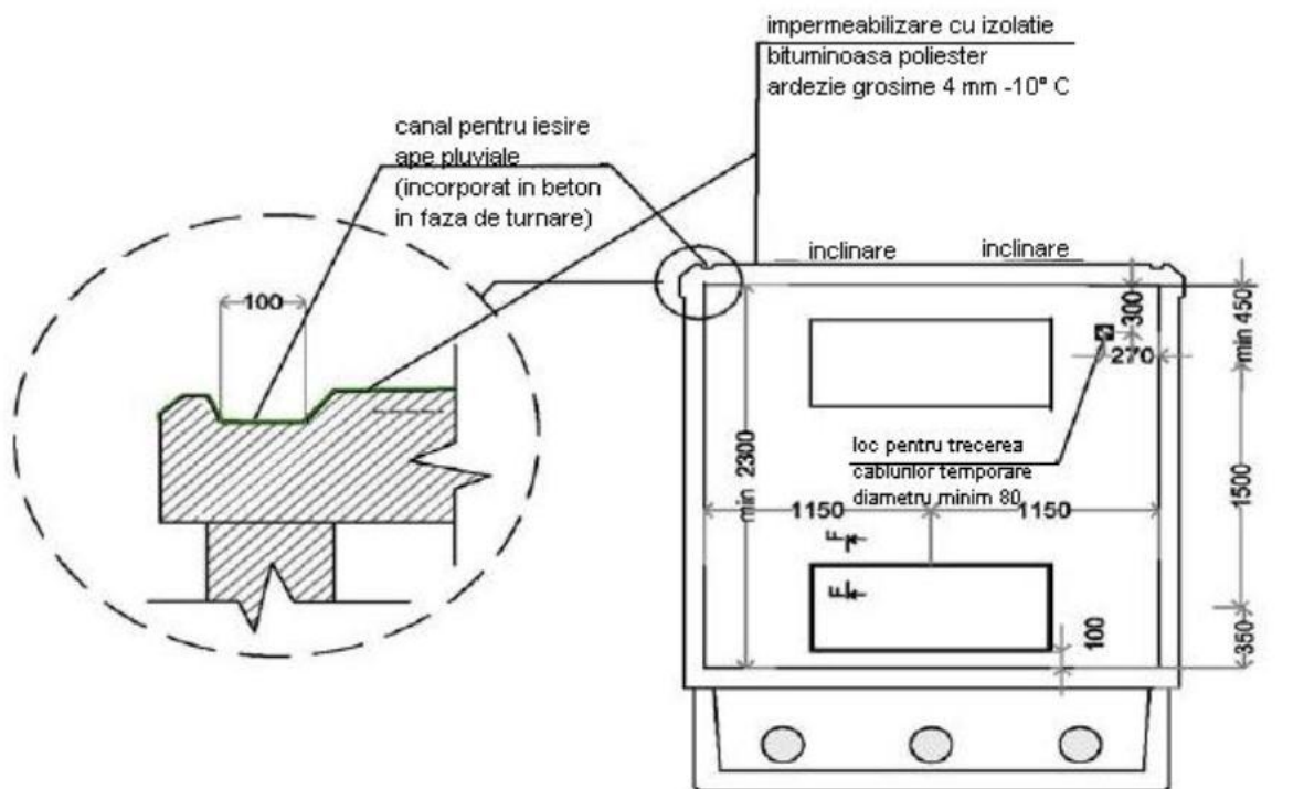
SECȚIUNE D-D
